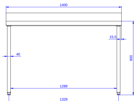
Boční
